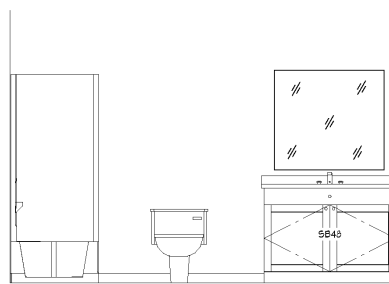
Bath Scale: 3/8"=1'
